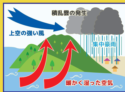
▲線状降水帯が発生するしくみ
